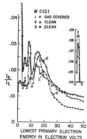
FIG. 10. I_b/I_t for tungsten (112).
